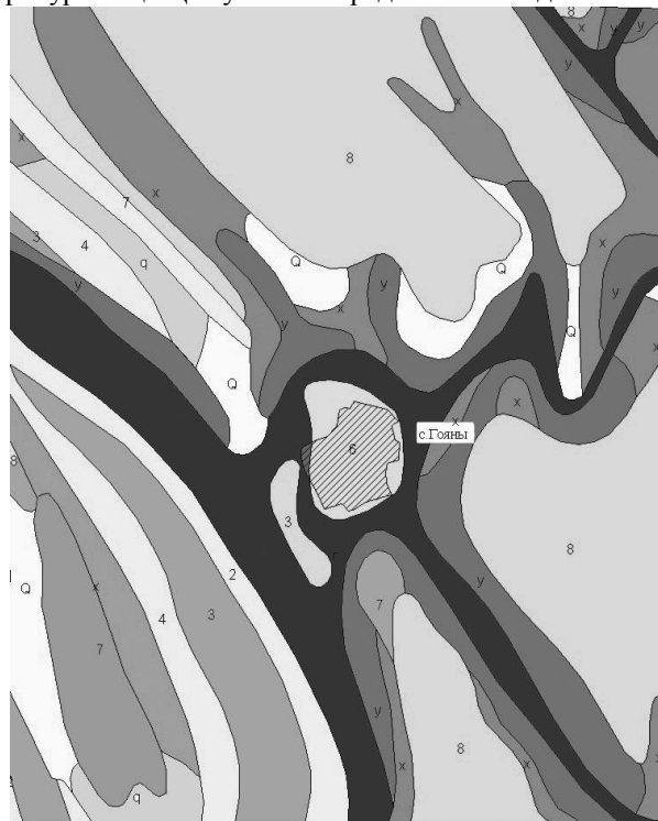
Рис. 2. Геоморфологические условия
