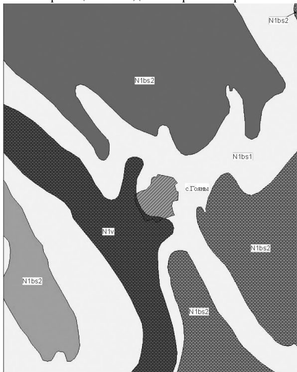
Рис. 1. Геологическое строение
